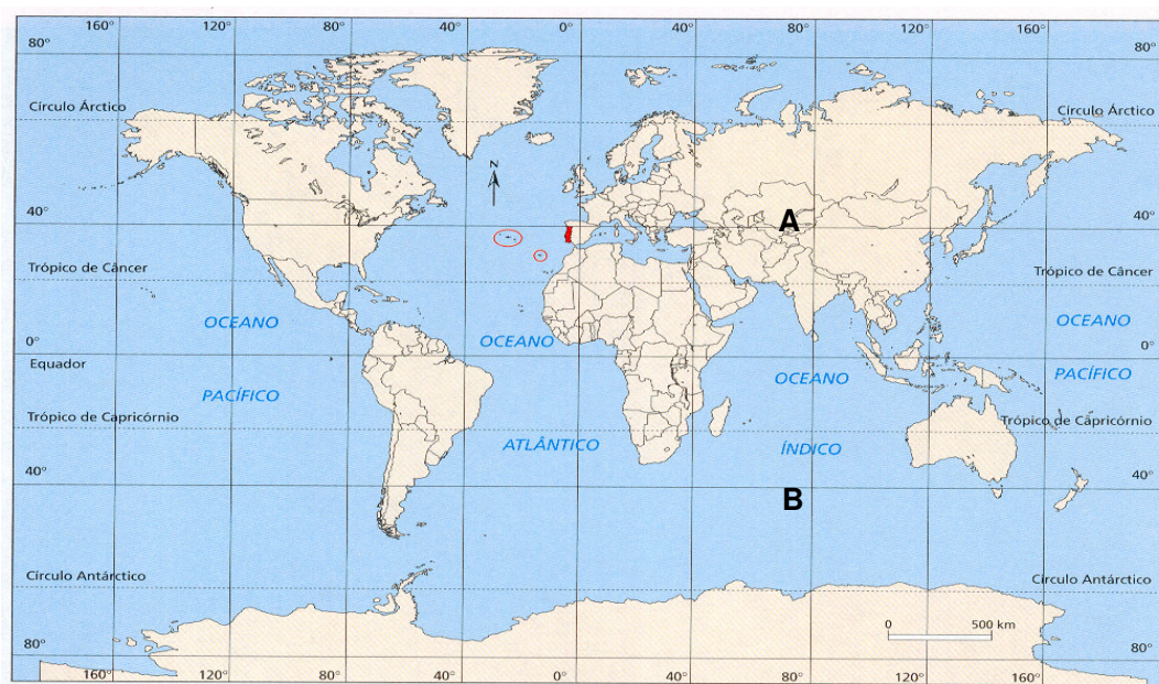
Fig. 1 – Planisfério
