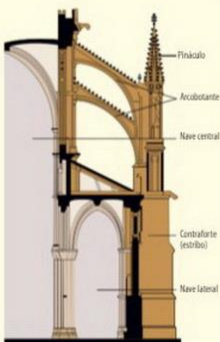
1. Corte esquemático.
