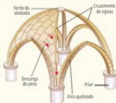
1. Esquema do tramo de uma abóbada de cruzamento de ogivas.
