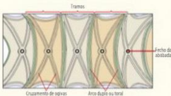
2. Abóbada de cruzamento de ogivas.
