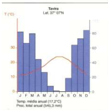
Imagem 2 – Gráfico Termopluviométrico
