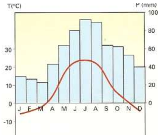
Imagem 4 – Gráfico termopluiométrico
